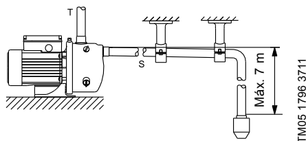
Fig. 2 Ligação à tubagem
