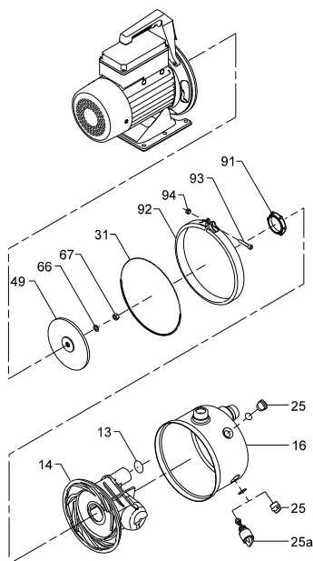
Рис. 6 Ежекторний насос у розібраному вигляді
