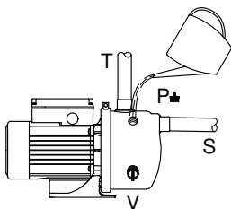
5. ilustr. Sūkņa piepildīšana ar ūdeni
