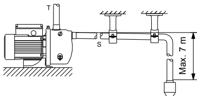
2. ábra Nyomócső csatlakoztatása
