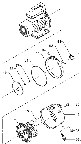
Fig. 6 Vista expandida da bomba ejectora
