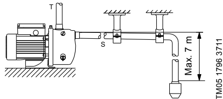
Slika 2 Povezivanje cevi
