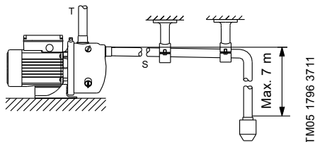
Slika 2 Cijevni priključci
