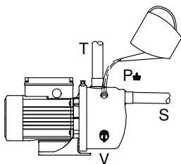
Рис. 5 Заповнення насосної установки водою
