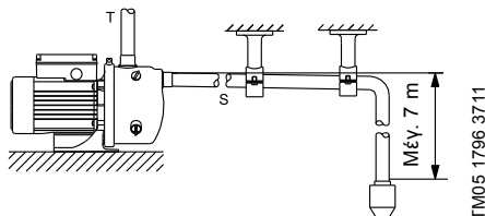
Σχ. 2 Σύνδεση σωλήνα
