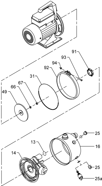
Şekil 6 Enjektörlü pompanın sökülüş halde görünümü
