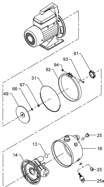
Σχ. 6 Αναλυτικό σχέδιο της αντλίας με τζιφάρι
