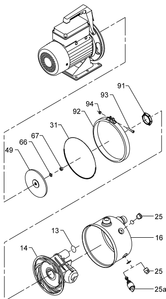
Kuva 6 Jet-pumpun hajotuskuva
