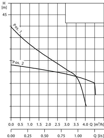
Fig. 3 Curva QH e posições da válvula do ejector
