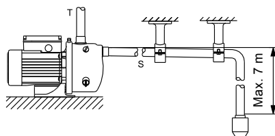
Afb. 2 Leidingaansluiting
