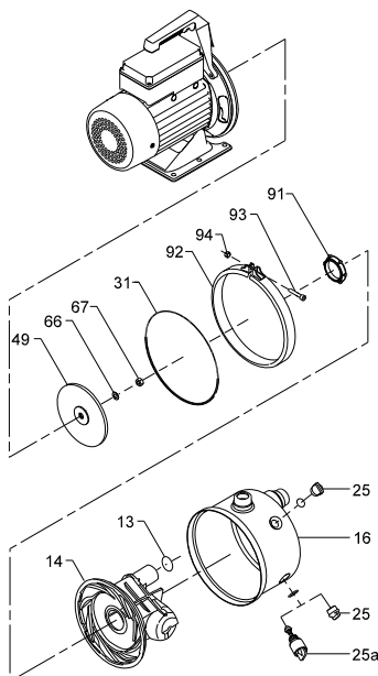
Fig. 6 Despiece de la bomba de chorro
