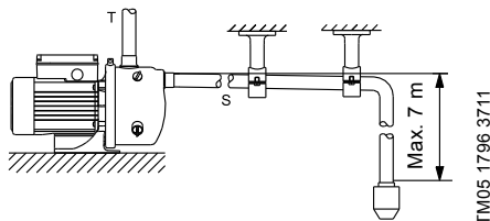
Fig. 2 Raccordement tuyauterie
