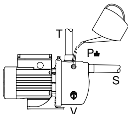
Slika 5 Punjenje crpke vodom
