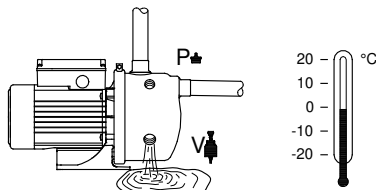
Slika 8 Sušenje črpalke
