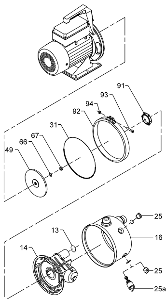
Фиг. 6 Детайлен изглед на джет помпа
