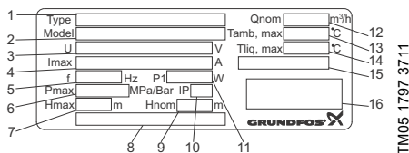
Fig. 1 Placa de características
