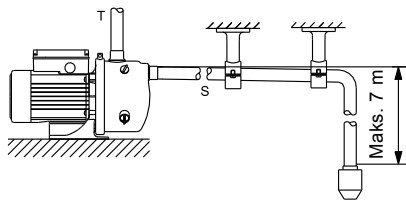
Kuva 2 Putkiliitäntä
