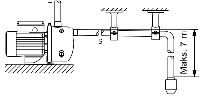
Şekil 2 Boru bağlantısı
