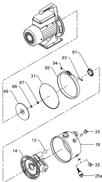
Fig. 6 Eksploderet tegning af jetpumpen
