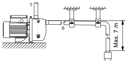
Abb. 2 Rohrleitungsanschluss
