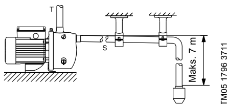
Fig. 2 Rørtilslutning
