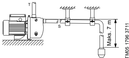
Slika 2 Cevni priključki
