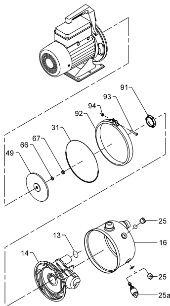
Slika 6 Sestavna risba Jet črpalke
